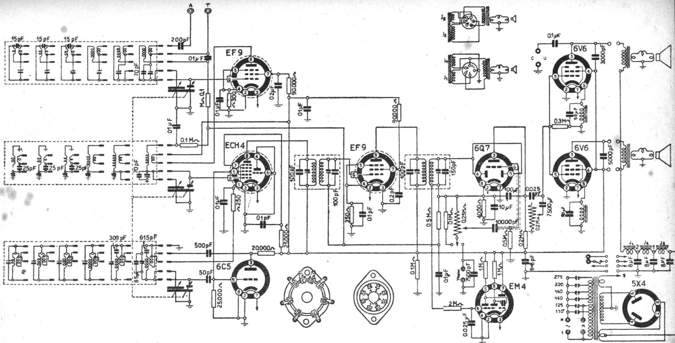
IMCA RADIO - Mod. IF 82 SERIE ESAGAMMA - Due gamme onde medie, quattro gamme onde corte: da 63,8 a 39,2 m, da 41,9 a 26,8 m, da 27,5 a 18,7 m, da 19,6 a 12,7 m. Potenza d'uscita: 8 W. Media frequenza: 467 kc/s.
